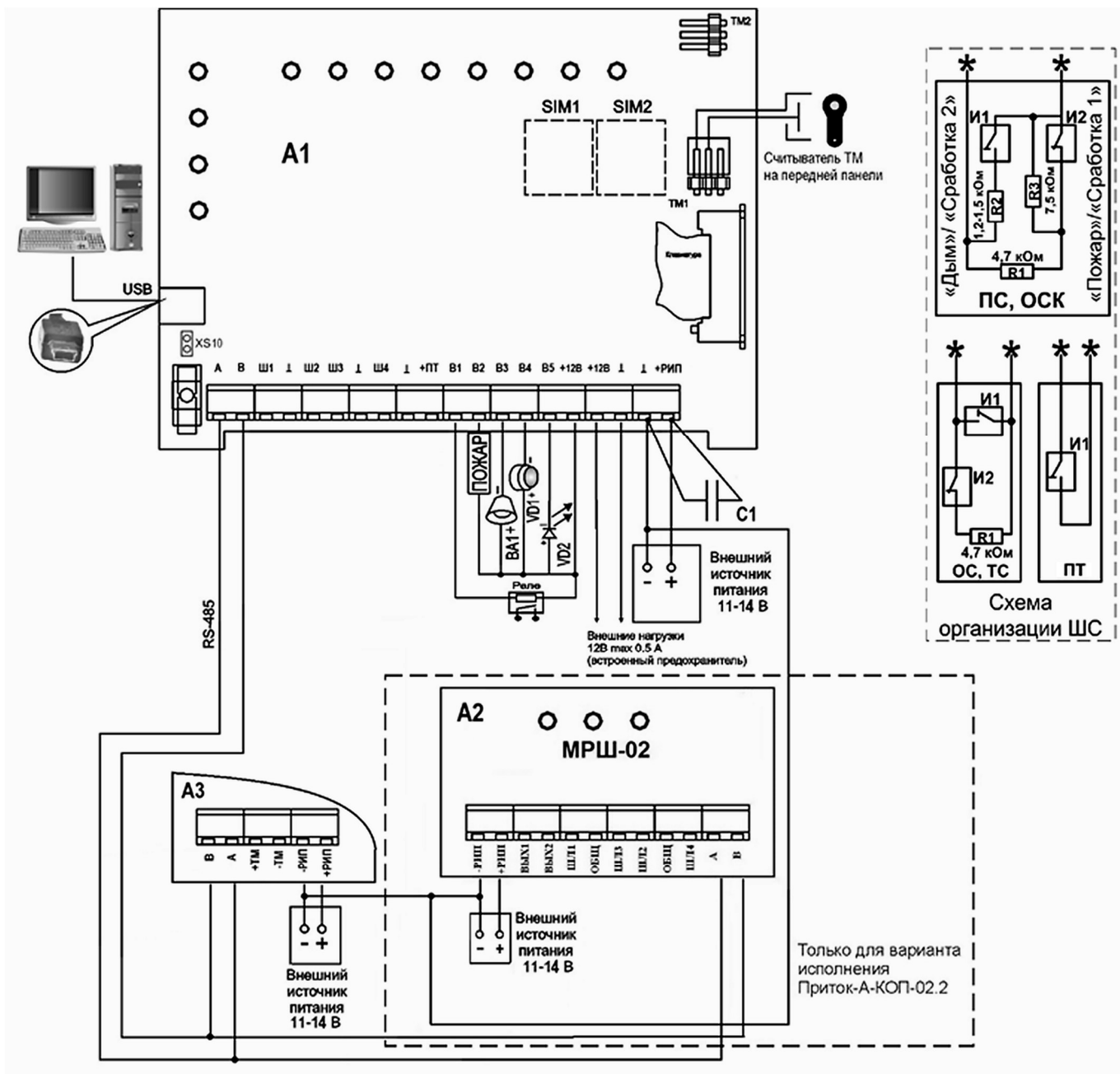
Рисунок 5 – Схема подключения
