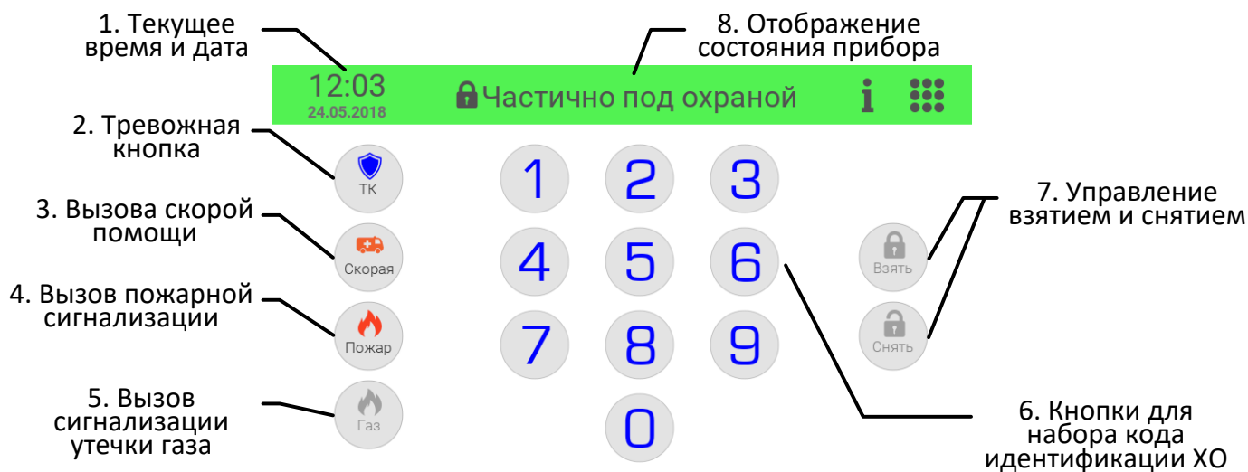
Рисунок 3 – Органы управления в режиме «Весь прибор»
