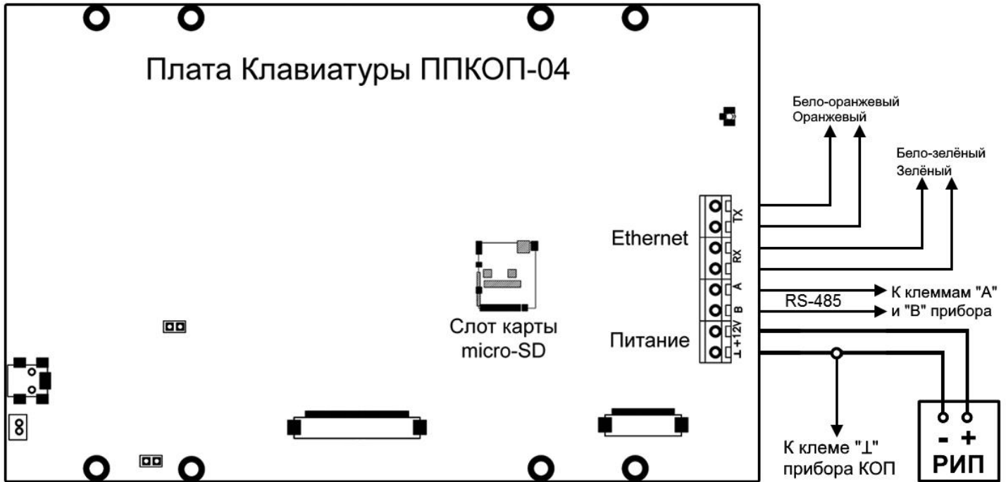
Рисунок 12 - Схема подключения клавиатуры к приборам серии Приток-А-КОП
